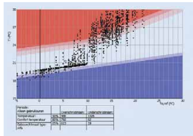
Case ATG31 – Normale ventilatiehoeveelheid; lokale koeling afwezig.
