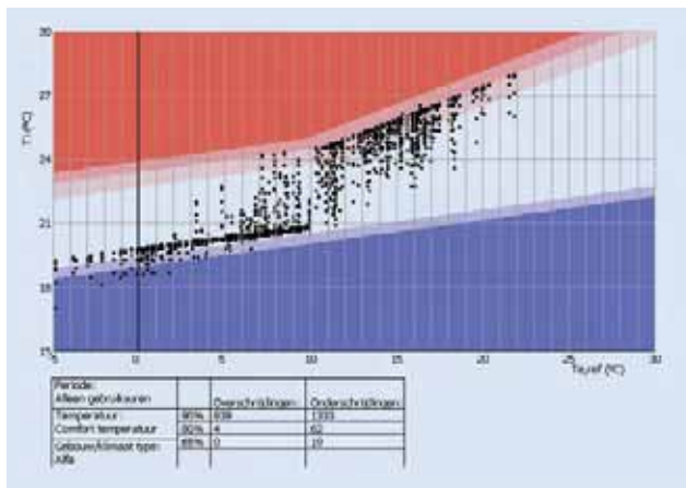
Case ATG31 – Normale ventilatiehoeveelheid; lokale koeling aanwezig.
