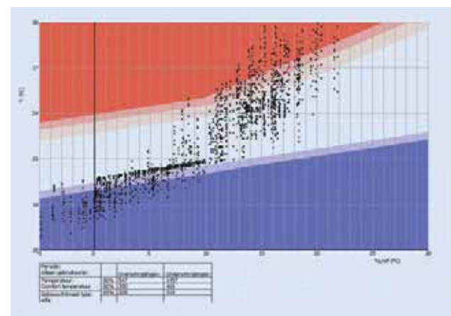
Case ATG32 – Dubbele ventilatiehoeveelheid; lokale koeling afwezig.
